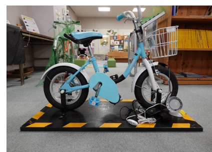
自転車発電機(幼児用)
